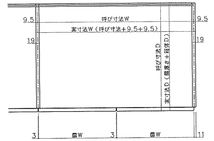
標準箱平面詳細図
