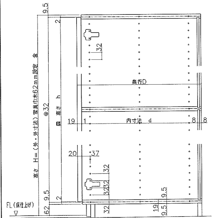
標準箱断面詳細図
